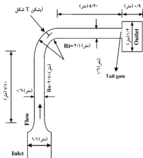
شکل ۲- کانال آزمایشگاهی.
