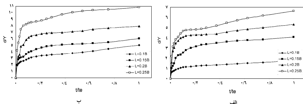
شکل ۹- تغییرات زمانی پیش‌روی چاله آب‌شستگی به سمت پایین‌دست، (الف): در موقعیت 30^\circ درجه و (ب): در موقعیت 60^\circ درجه.
