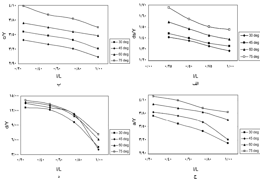
شکل ۱۷- تغییرات ابعاد حفره آب شستگی نسبت به طول بال آب شکن در پایان زمان تعادل و در موقعیت های مختلف استقرار آب شکن، (الف): عمق آب شستگی حداکثر (ب): پیش روی حفره به سمت بالادست (ج): پیش روی حفره در عرض کانال (د): پیش روی حفره به سمت پایین دست.
