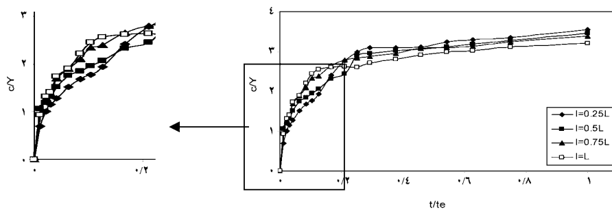
شکل ۱۱- تغییرات زمانی پیش‌روی چاله آب‌شستگی به سمت بالادست آب‌شکن برای طول‌های مختلف بال آب‌شکن در موقعیت ۳۰ درجه.
