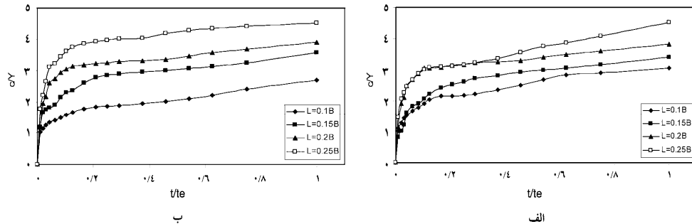
شکل ۷- تغییرات زمانی پیشروی چاله آب‌شستگی به سمت بالادست برای طول‌های مختلف، (الف): در موقعیت ۳۰ درجه و (ب): در موقعیت ۶۰ درجه.
