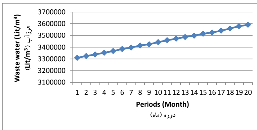
شکل ۵- مقادیر حاصل از هرزآب در ابعاد مختلف.
