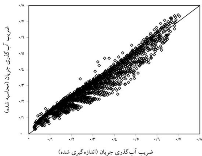
شکل ۲- تغییرات ضریب آب گذاری محاسبه شده از رابطه ۱۳ در برابر مقادیر مشاهده شده.
