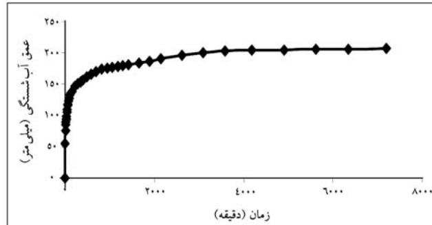
شکل ۲- تغییرات زمانی عمق آبستگی در آزمایش زمان تعادل.
