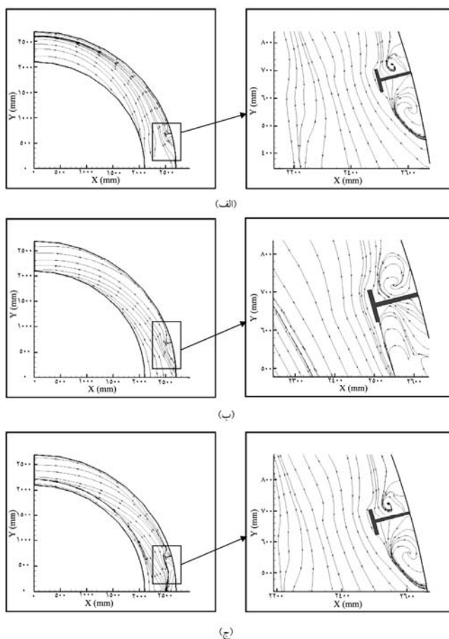
شکل ۱۴- نمونه‌ای از الگوی جریان در پلان‌های مختلف قوس ۹۰ درجه با آب‌شکن مستقر در زاویه ۷۵ درجه و بستر تعادل‌یافته در بالای چاله آب‌شستگی در فاصله از بستر اولیه (الف) ۵ میلی‌متر، (ب) ۶۰ میلی‌متر و (ج) ۱۱۵ میلی‌متر.
