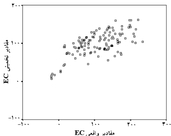
شکل ۴- نمودار پراکنش مقادیر واقعی و تخمین زده شده هدایت الکتریکی سطحی.
