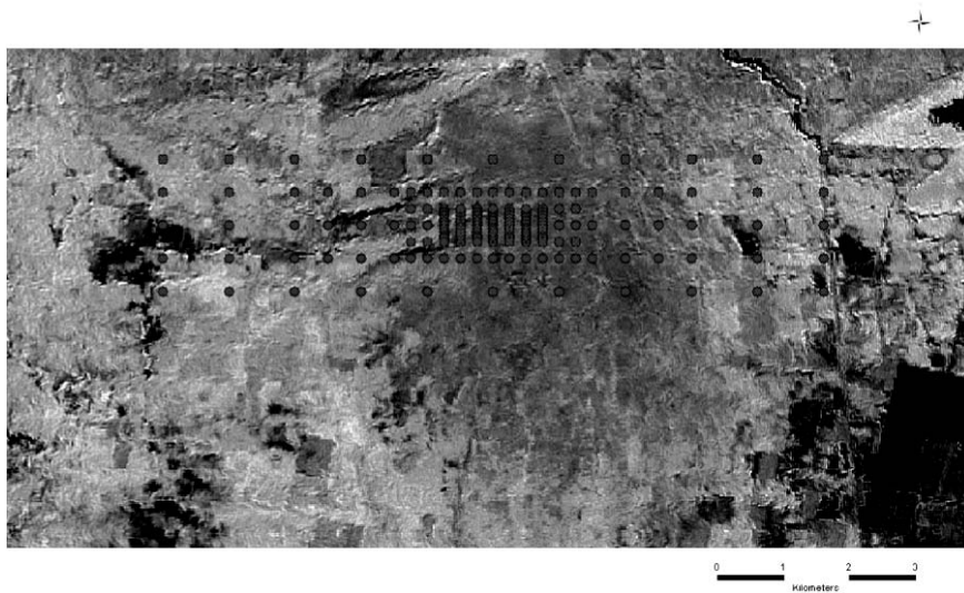
شکل ۲- محل نقاط نمونه‌برداری در منطقه مورد مطالعه بر روی تصویر ETM^+
