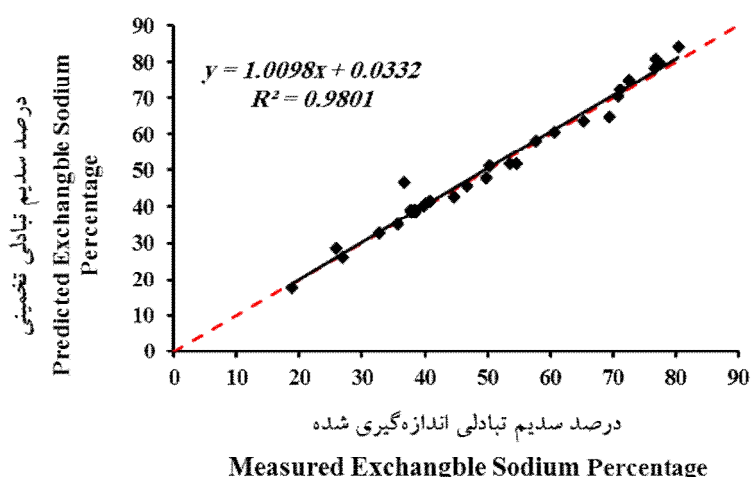
شکل ۵- مقادیر درصد سدیم تبادلی تخمینی و اندازه‌گیری شده با استفاده از مدل شبکه بیزین. Figure 5. Correlation of predicted and measured ESP by Bayesian network model.
