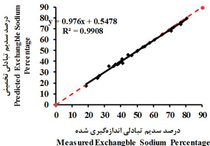
شکل ۴- رابطه بین درصد سدیم تبادلی تخمینی و اندازه‌گیری شده با مدل حداقل مربعات معمولی.
