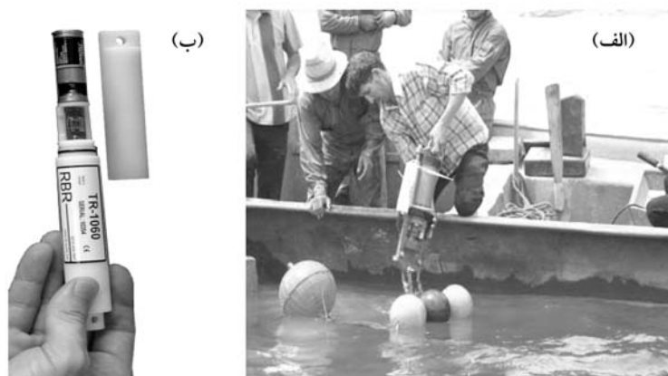
شکل ۸- نمایی از دستگاه‌های جریان‌سنج (الف) و کدورت‌سنج (ب).
