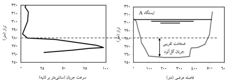
شکل ۱۱- تعیین ضخامت و عرض لایه جریان گل‌آلود در ایستگاه A با استفاده از اندازه‌گیری‌های صحرائی.
