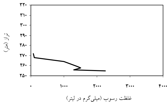
شکل ۱۲- پروفیل قائم تغییرات غلظت رسوب در ایستگاه A با استفاده از اندازه‌گیری‌های صحرایی (بی‌نام، ۲۰۰۴).
