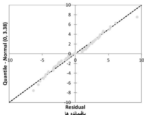
شکل ۲۴- نمودار Q-Q باقی‌مانده‌های رگرسیون خطی معمولی (تداوم). Figure 24. Q-Q plot residuals of OLR (Duration).
