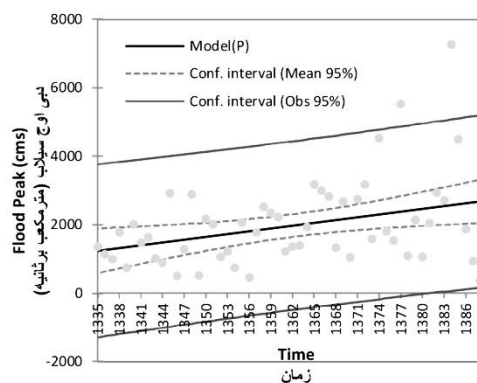
شکل ۱- برازش مدل رگرسیون خطی معمولی (دبی اوج).
