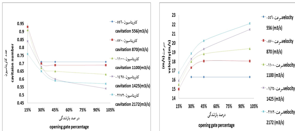
شکل ۶- سرعت و کاویتاسیون در بازشدگی‌های ۱۵، ۳۰، ۴۵ و ۱۰۰ در ۵ دی در ابتدای پرتاب‌کننده.
