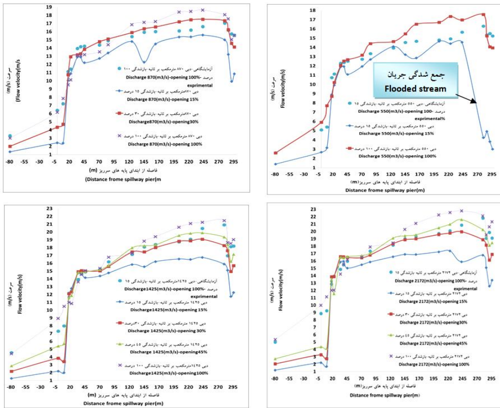
شکل ۵- مقایسه سرعت جریان در طول سرریز، در بازشدگی‌های ۱۵، ۳۰، ۴۵ و ۱۰۰ درصد در ۴ دی.
