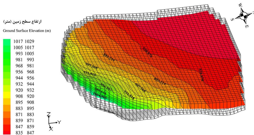
شکل ۶- شکل هندسی آبخوان دشت روداب.
