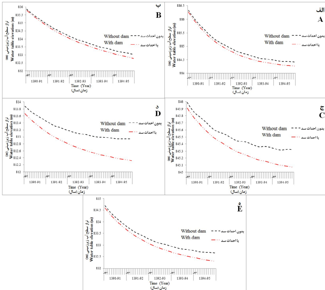
شکل ۱۵- مقایسه هیدروگراف پیش‌بینی سطح آب مشاهده‌ای در شرایط وجود و نبود سد روداب در چاه‌های مشاهده‌ای (الف) تسبند (ب) فیلشور (ج) جنوب کال برآباد (د) قلعه‌نو ملوند (ه) دروک.
