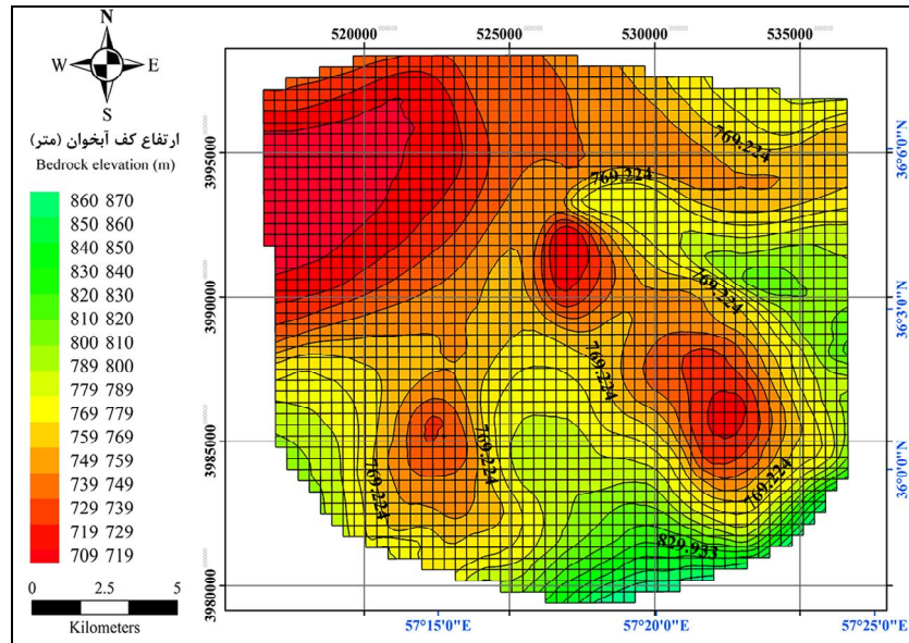
شکل ۵- توپوگرافی سنگ بستر آبخوان دشت روداب.
