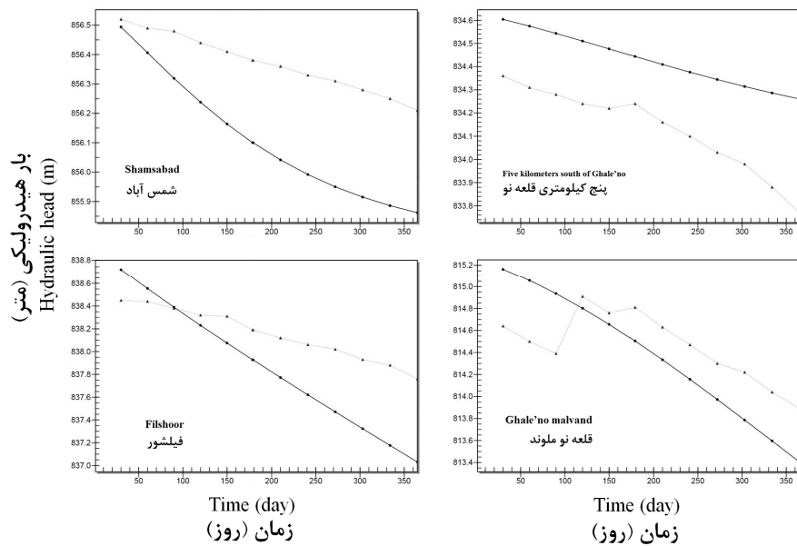
شکل ۹- مقایسه هیدروگراف سطح آب مشاهده‌ای نسبت به محاسبه‌ای در چاه‌های مشاهده‌ای (پنج کیلومتری جنوب قلعه‌نو، شمس‌آباد، قلعه‌نو ملوند، فیلشور).
