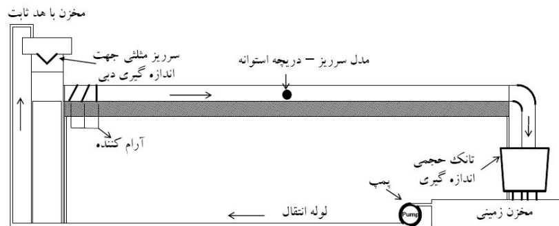
شکل ۱- شکل و اجزای فلوم آزمایشگاهی مورد استفاده.
