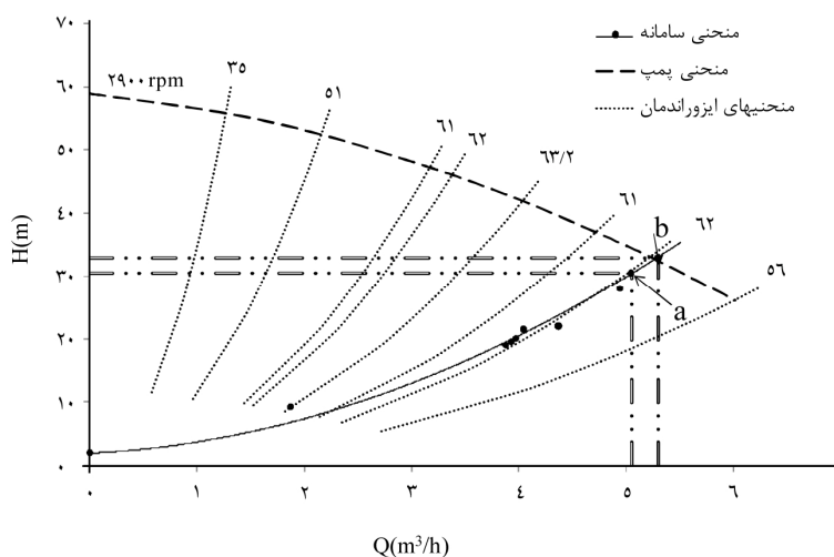
شکل ۱- منحنی سامانه و نقاط عملکرد ایده‌آل و طراحی شده در شرایط حداکثر نیاز آبی سامانه تحت فشار نمونه.
