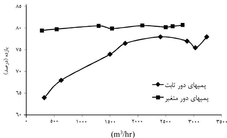
شکل ۱۰- نمودار تغییر بازده هر پمپ، در دوره‌های مختلف آبیاری در طول سال، در دو حالت تنظیم ایستگاه پمپاژ.
