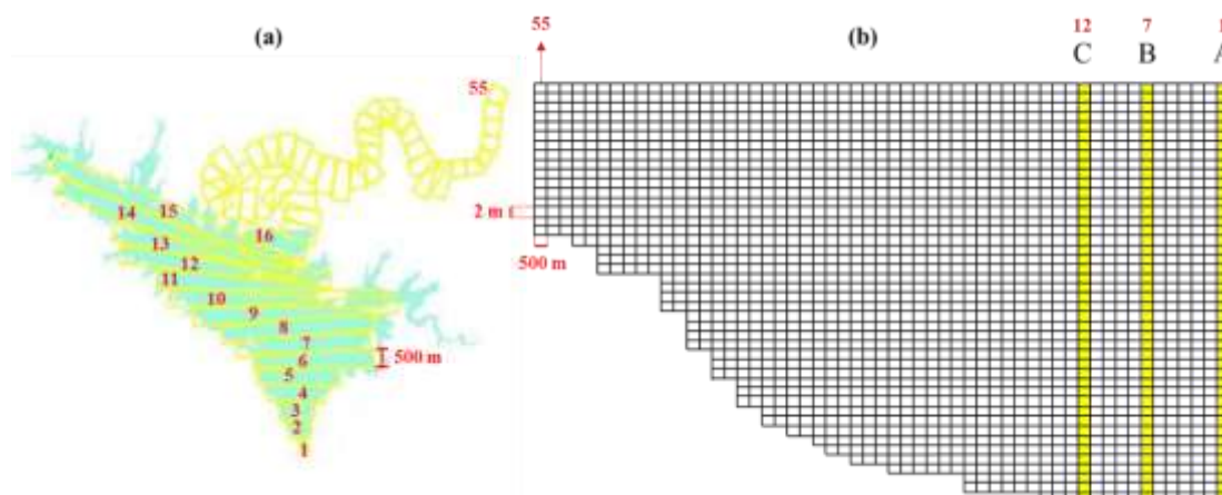
شکل ۲- موقعیت بخش‌های حاصل تقسیم‌بندی دریاچه سد دز و رودخانه منتهی به آن و ایستگاه‌های اندازه‌گیری پروفیل دمایی آب مخزن: (الف) دید از بالا، و (ب) نمای جانبی.
