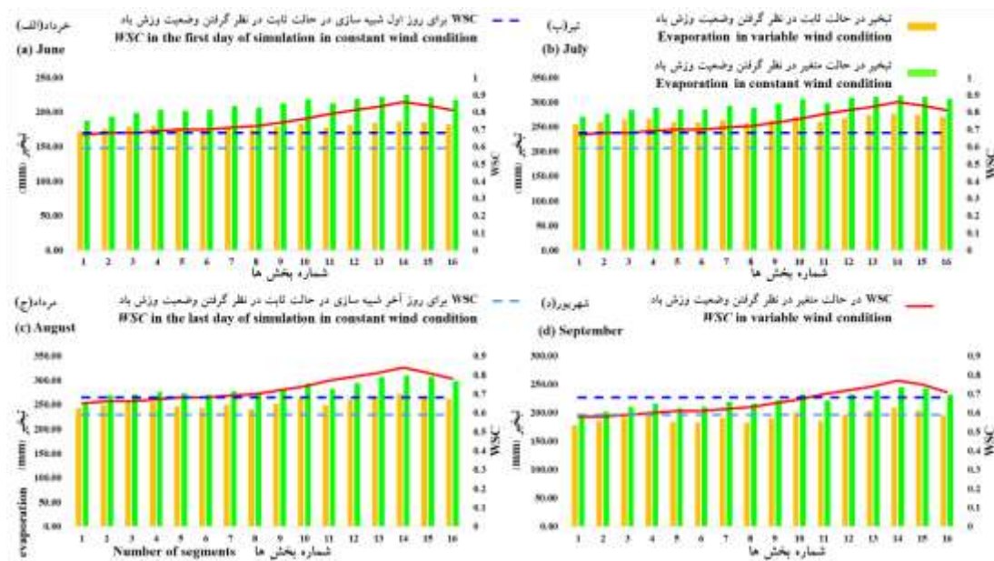
شکل ۵- مقایسه تبخیر ماهانه برآورد شده در دو حالت ثابت و متغیر در نظر گرفتن وضعیت باد، به تفکیک هر یک از بخش‌های دریاچه و ماه‌های خرداد، تیر، مرداد و شهریور.
