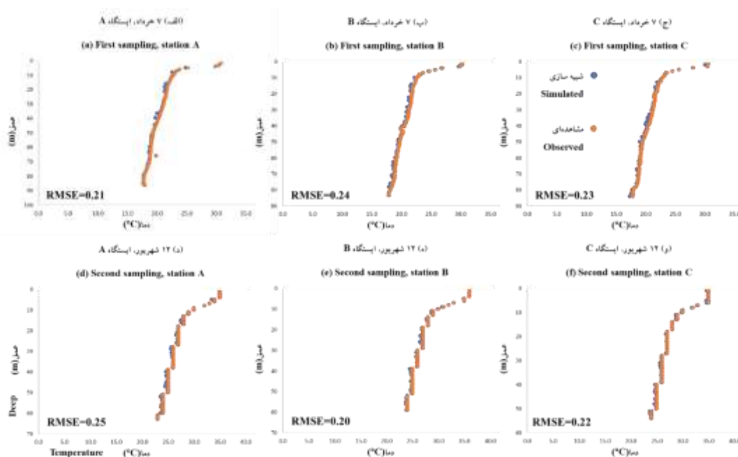
شکل ۴- پروفیل‌های حرارتی شبیه‌سازی شده و اندازه‌گیری شده در روزها و ایستگاه‌های نمونه‌برداری، در حالی که شرایط باد متغیر در نظر گرفته شده است.
