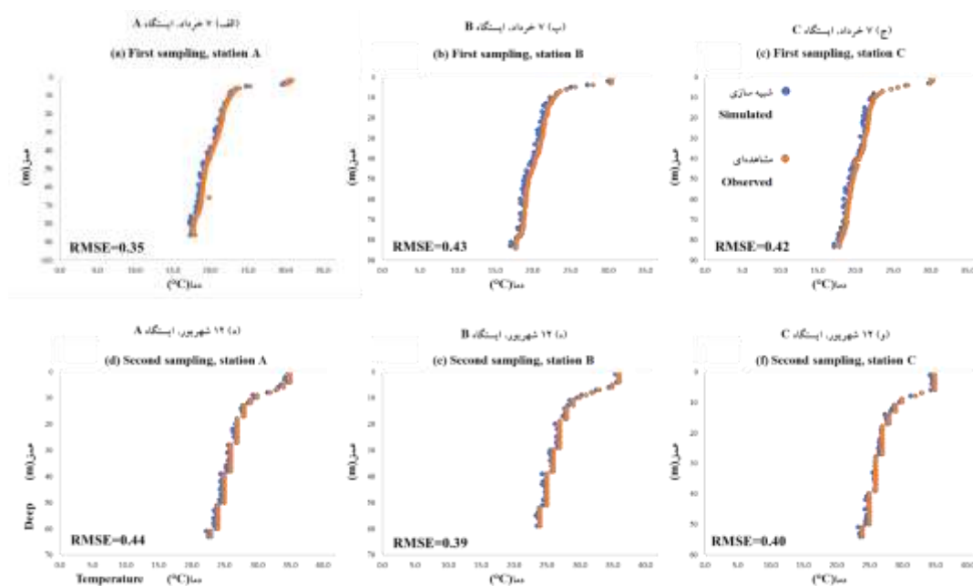
شکل ۳- پروفیل‌های حرارتی شبیه‌سازی و اندازه‌گیری شده در روزها و ایستگاه‌های نمونه‌برداری، در حالت ثابت در نظر گرفتن باد در تمام بخش‌های دریاچه.
