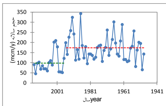
شکل ۳- آزمون پتی حجم جریان سالانه در ایستگاه بند.
