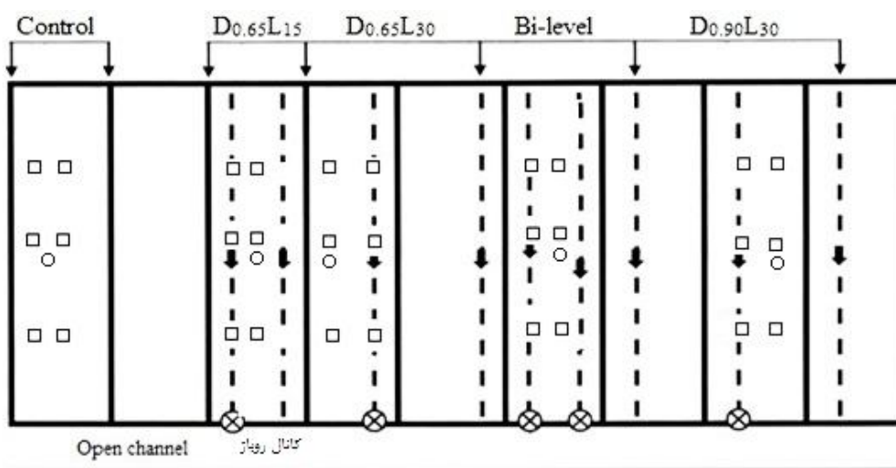
شکل ۱- آرایش سیستم‌های زهکشی در مزرعه مورد مطالعه (محل نمونه برداری، \square چاهک سطح ایستابی، \otimes خروجی زهکش، مرکز کرت، \leftarrow خطوط زهکش).
