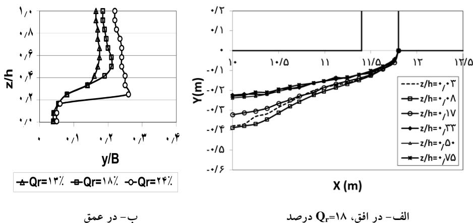
شکل ۵- تغییرات خط جدایی جریان با نصب صفحات مستغرق.
