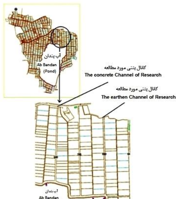
شکل ۳- جانمایی کانال های مورد مطالعه در پروژه تجهیز و نوسازی اراضی شالیزاری اسماعیل کلا. Figure 3. Location of Studied channels in Esmaekola paddy fields renovation project.
