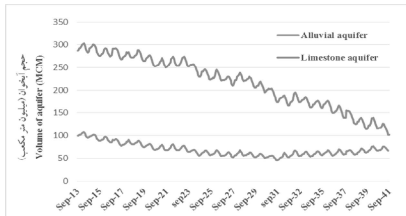
شکل ۷- حجم آبخوانهای آبرفتی و آهکی طی سالهای شبیه‌سازی برای سناریو S 21 .
