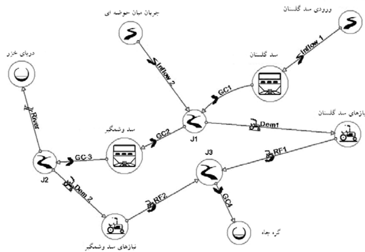
شکل ۲- شماتیک مدل ساخته شده برای سیستم دو سد گلستان و وشمگیر.
