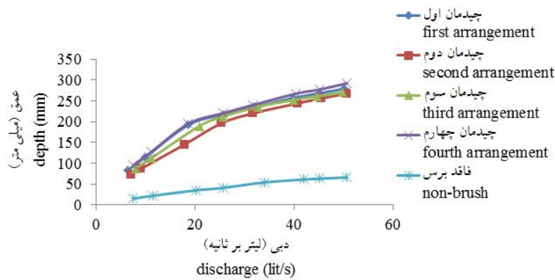
شکل ۷- منحنی دبی- عمق برای چیدمان‌های مختلف در شیب ۲٪.
