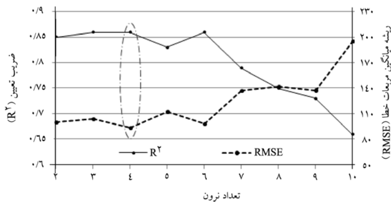
شکل ۳- اثر تعداد نرون‌های لایه پنهان بر روی شاخص‌های R^2 و RMSE برای مدل NN-1-TV.
