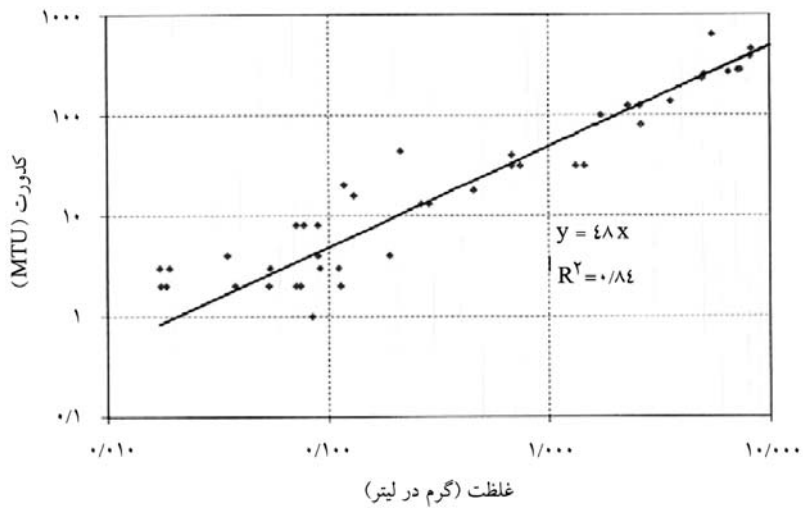
شکل ۱۰- رابطه کدورت- غلظت رسوب معلق در مخزن سد دز در ایستگاه F (بی‌نام، ۲۰۰۴).
