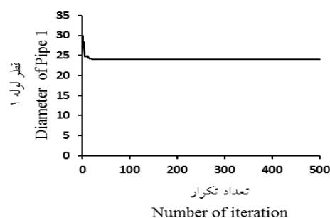
شکل ۵- تغییرات قطر لوله ۱ در مقابل تعداد تکرار.
