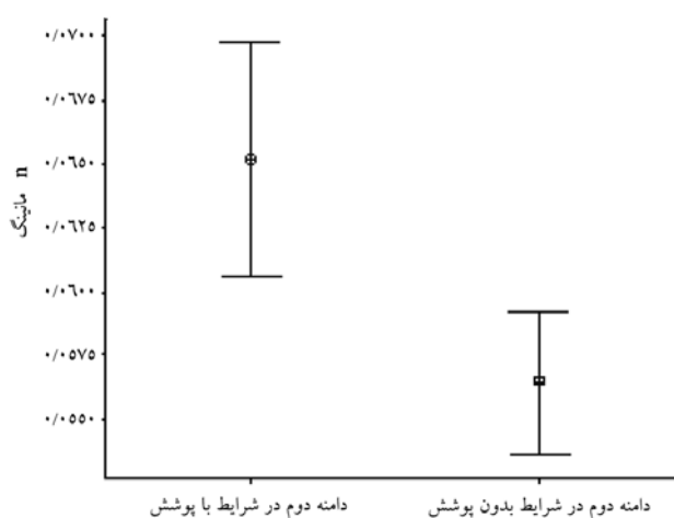
شکل ۱۰- پلات میانگین ضریب مانینگ برای دامنه با شیب ۱۲/۹ درصد.
