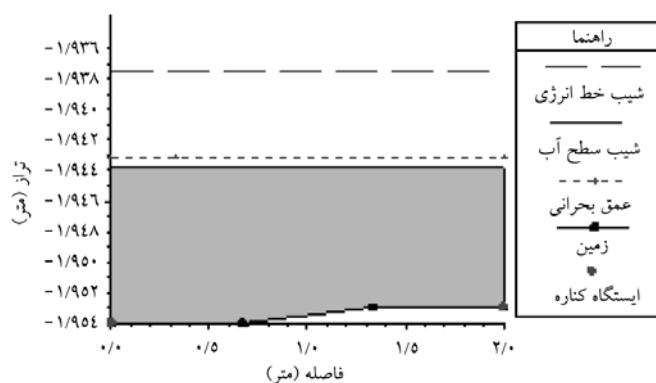
شکل ۷- مقطع عرضی ۲، بدون پوشش، شیب ۱۲/۹ درصد، تکرار ۵.
