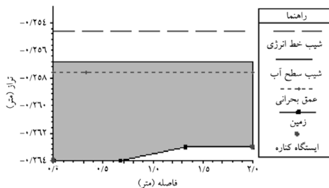
شکل ۶- مقطع عرضی ۵، بدون پوشش، شیب ۴/۱ درصد، تکرار ۵.
