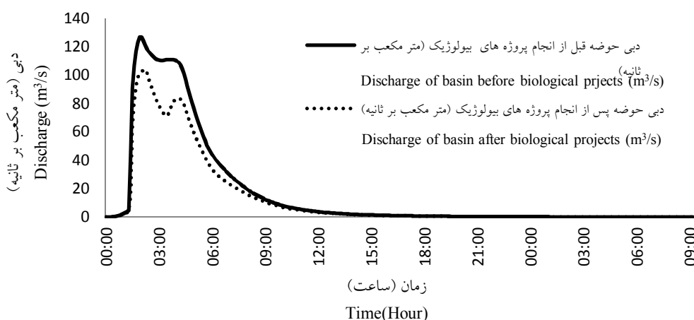
شکل ۱۰- نمودار تأثیر پروژه‌های بیولوژیک بر هیدروگراف سیل حوضه (دوره بازگشت ۱۰۰ ساله).
