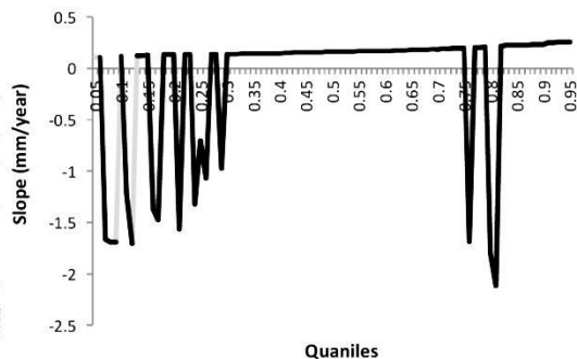
شکل ۱۸- نمودار تغییرات شیب خط رگرسیون کوانتایل (ارومیه). Figure 18. Plot of slope of quantile regression lines (Urmia).
