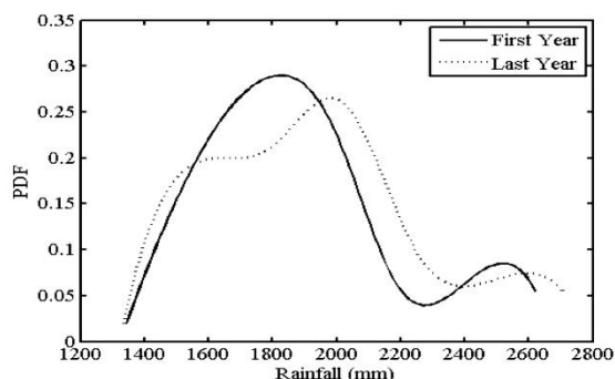
شکل ۱۳- نمودارهای EPDF در ابتدا و انتهای دوره (بندرانزلی).
