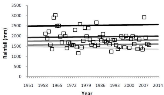
شکل ۱۱- نمودار خطوط رگرسیون کوانتایل (بندرانزلی).
