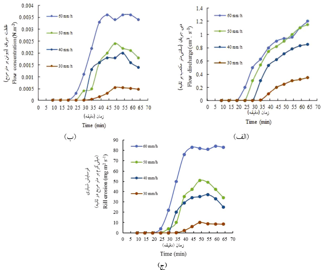
شکل ۱- رابطه بین زمان و دبی جریان (الف)، غلظت جریان (ب) و فرسایش شیاری (ج) در شدت‌های مختلف باران در خاک مارنی.
