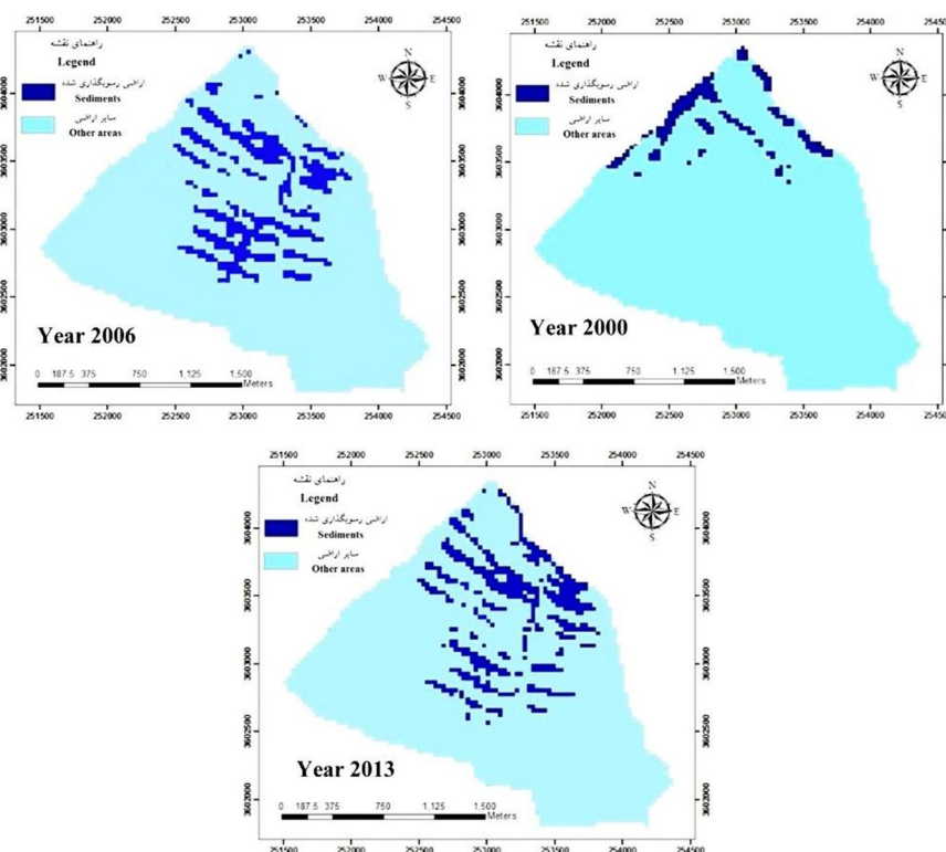
شکل ۲- محدوده‌های رسوبگذاری در عرصه پخش سیلاب در پایان هر دوره.
