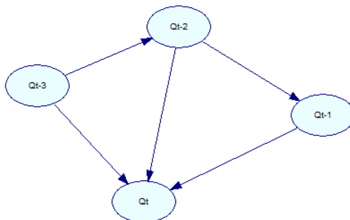
شکل ۲- مدل مفهومی ساخته شده برای شبکه بی‌زین. Figure 2. Bayesian networks conceptual model.
