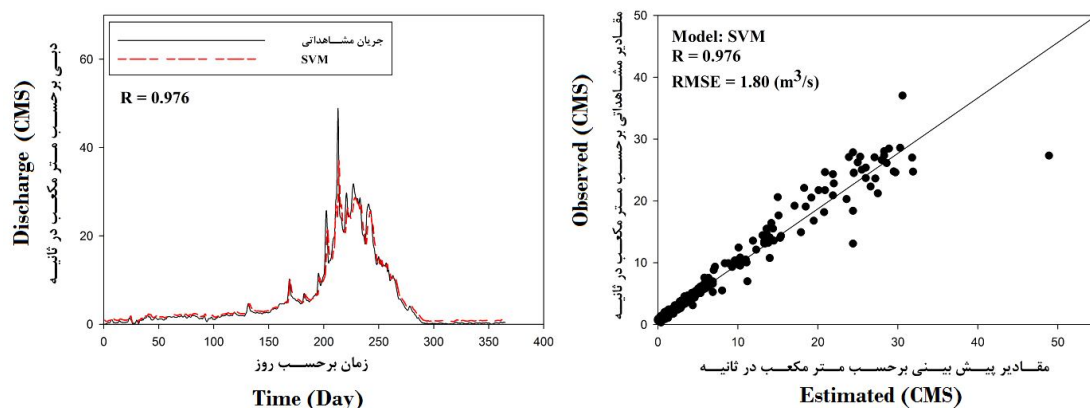
شکل ۴- نمودارهای مقادیر مشاهده‌ای و مقادیر پیش‌بینی شده حاصل از مدل SVM در مرحله صحت‌سنجی.
