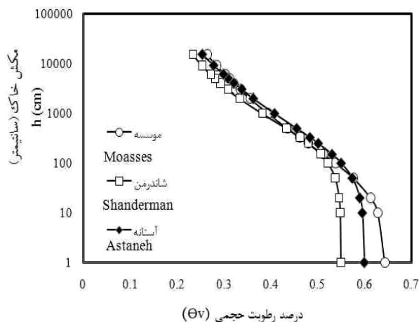
شکل ۲- منحنی مشخصه رطوبتی در خاک‌های مورد مطالعه (20).
