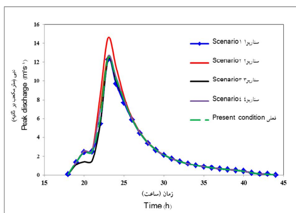
شکل ۵- اثر سناریوها بر هیدروگراف سیل واقعه ۱ و ۲ و ۱۳۷۶/۸/۲۳.
