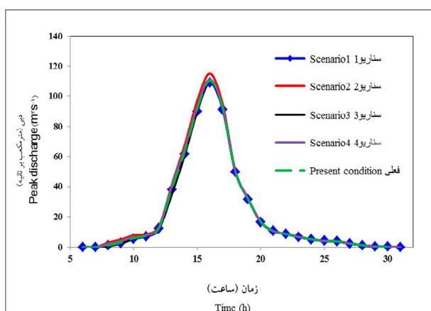
شکل ۶- اثر سناریوها بر هیدروگراف سیل واقعه ۳۰ و ۳۱ و ۱۳۸۴/۲/۲۰.
