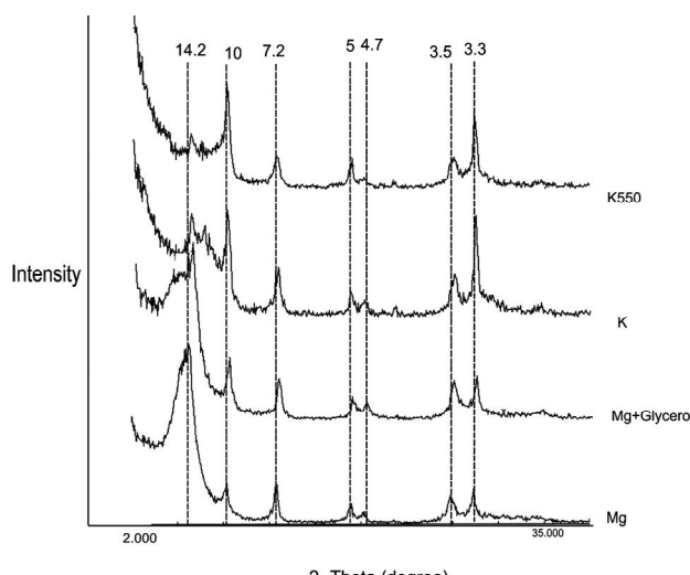
شکل ۱- دیاگرام کانی‌شناسی جزء رس نمونه خاک شماره ۸
