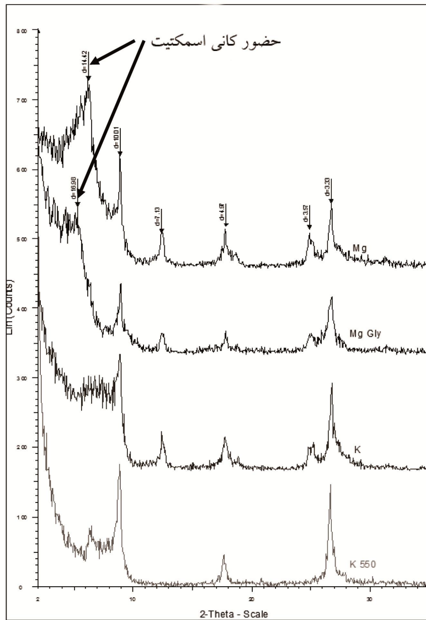
شکل ۳- پرتونگاری اشعه ایکس بخش رس، پیک 17\text{\AA} در تیمار گلیسرول نشان‌دهنده کانی اسمکتیت می‌باشد (سری خاک قره‌سو، افق A_p ).
