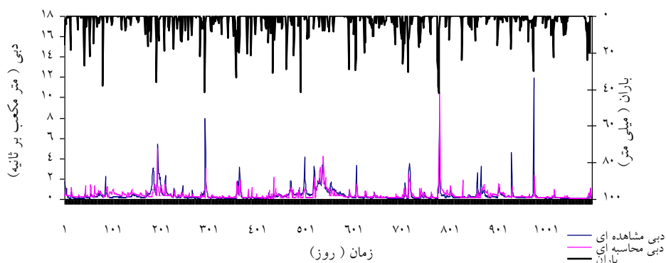
شکل ۱- دبی روزانه مشاهده‌ای و شبیه‌سازی شده روزانه مدل WetSpa برای دوره آزمون.
