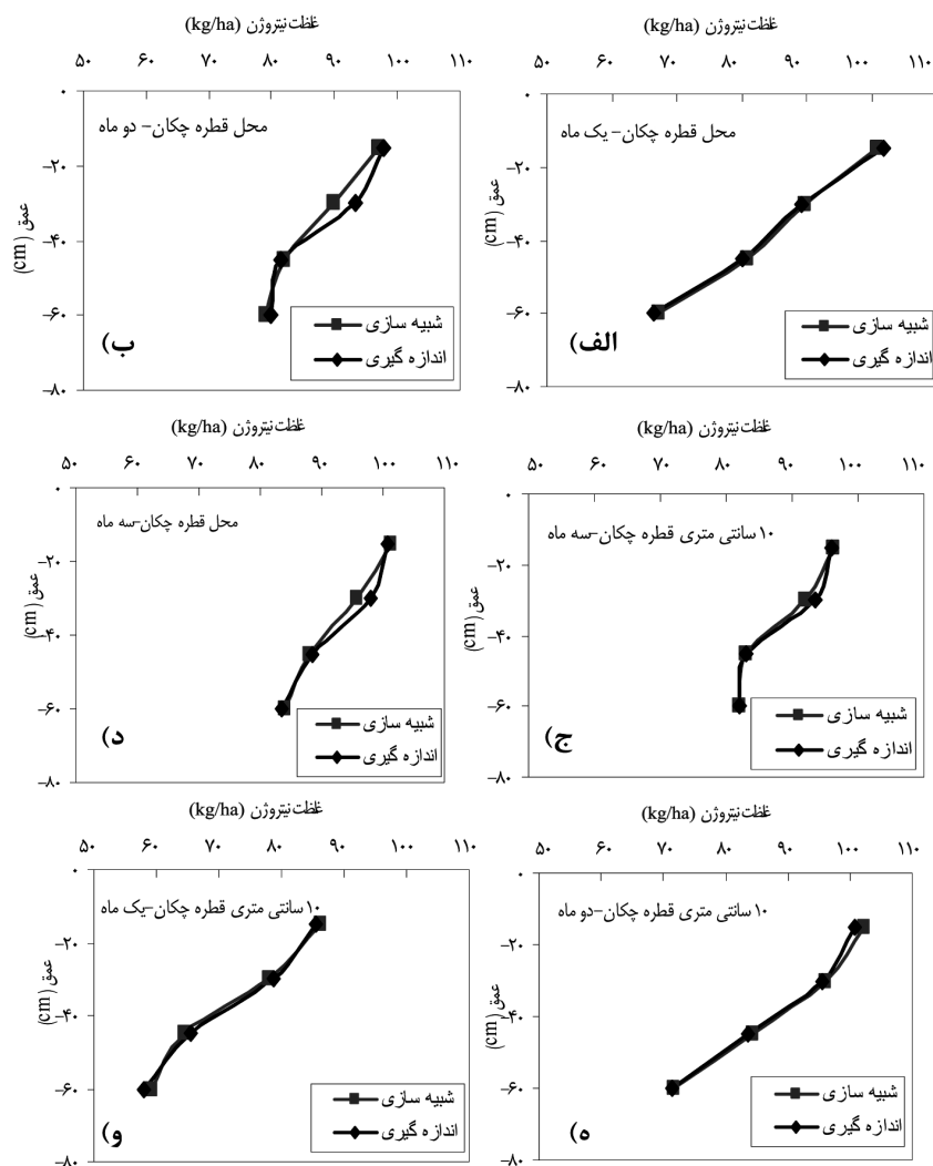
شکل ۲- شبیه‌سازی الگوی توزیع نیتروژن تا عمق ۶۰ سانتی‌متر ۱، ۲ و ۳ ماه پس از نشاء.
