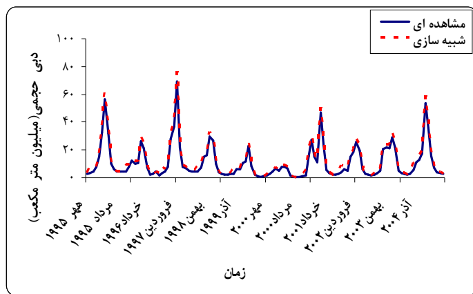
شکل ۷- مقایسه حجم مخزن فارسان-جوققان در دو حالت مشاهده‌ای و شبیه‌سازی.
