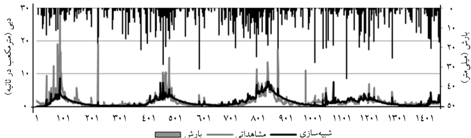
شکل ۱- هیدروگراف شبیه‌سازی شده پس از واسنجی مدل (۲۰۰۱-۲۰۰۴).
