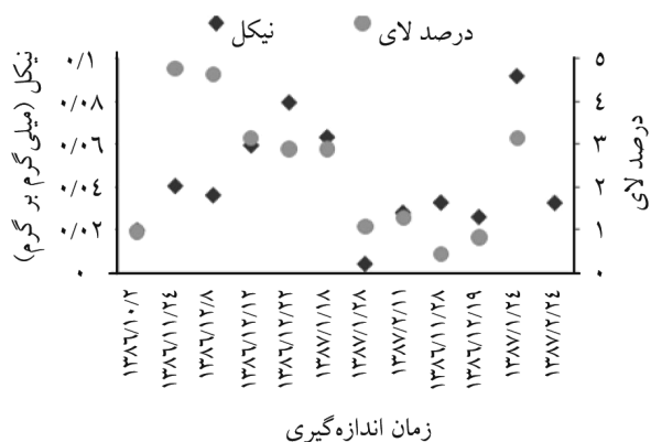
شکل ۶- الگوی تغییرات نیکل و درصد لای در پایین دست. زمان اندازه گیری
