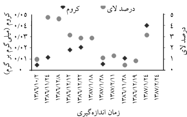
شکل ۷- الگوی تغییرات کروم و درصد لای در پایین دست. زمان اندازه گیری
